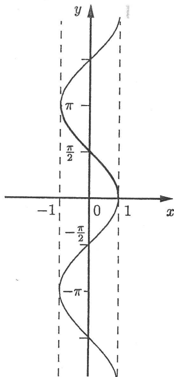
Abbildung 6.18 Arkuskosinuskurve
