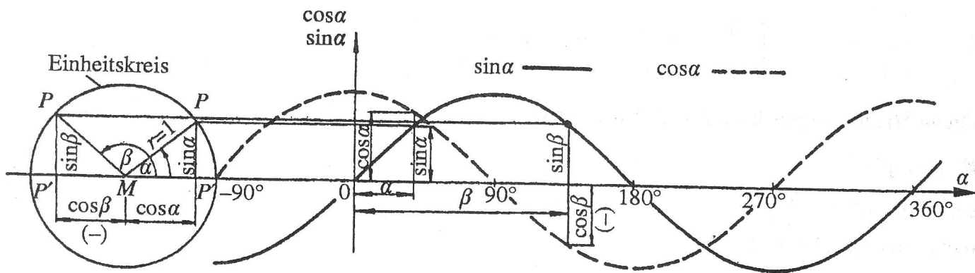
Abbildung 6.7 Sinuskurve und Kosinuskurve
