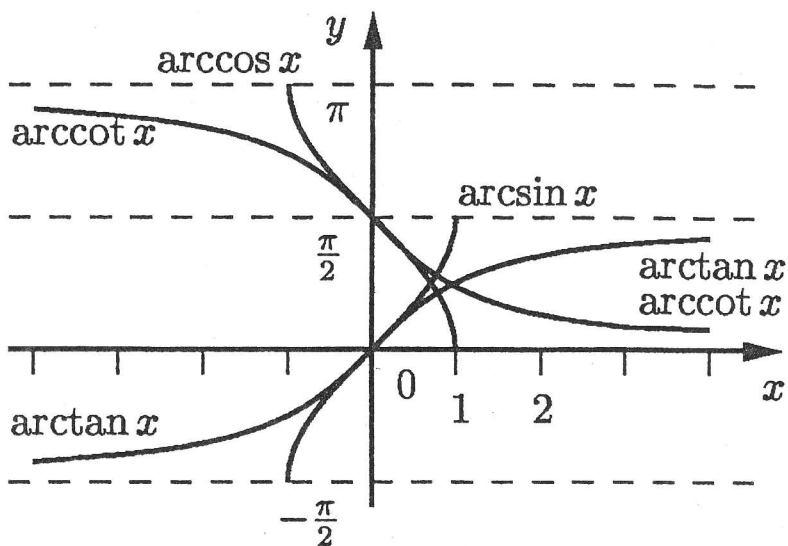
Abbildung 6.21 Hauptwerte der Arkusfunktionen
