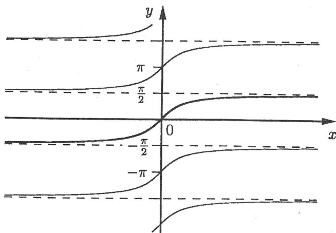
Abbildung 6.19 Arkustangenskurve
