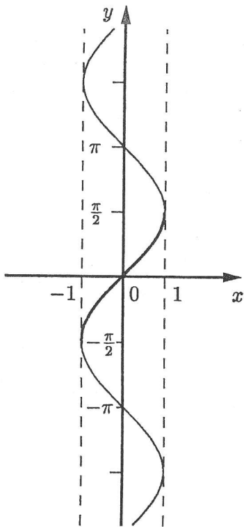
Abbildung 6.17 Arkussinuskurve
