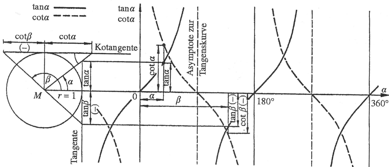
Abbildung 6.8 Tangenskurve und Kotangenskurve
