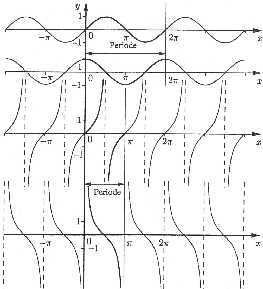
Abbildung 6.9 y = \sin x , y = \cos x , y = \tan x , y = \cot x (von oben nach unten)
